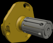
Spanndorn Größe 2-4 Ø32 -90 mm
